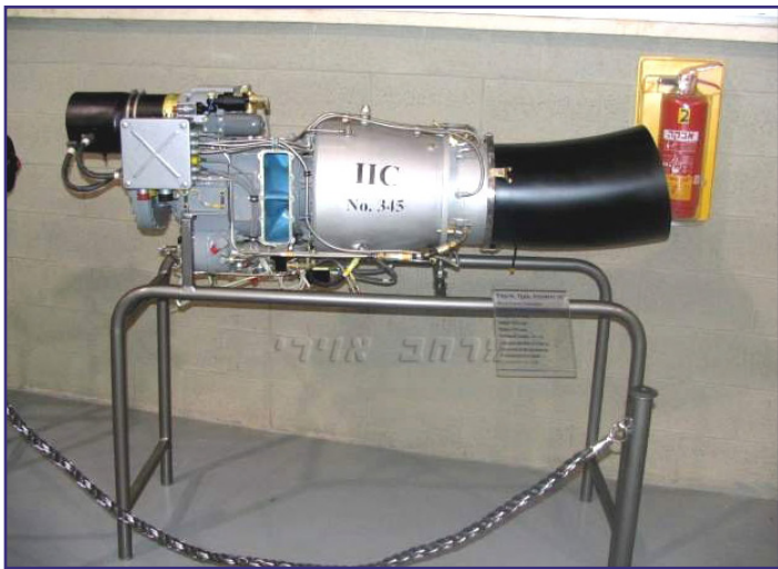
מנוע ארטוסט-מסוק אלואט.
