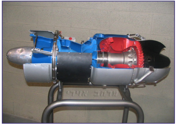
חתך מנוע שורק 4.
