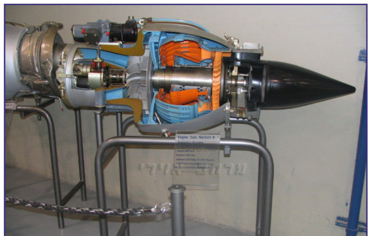
חתך מנוע מרבורה -2 מטוס פוגה מגיסטר.
