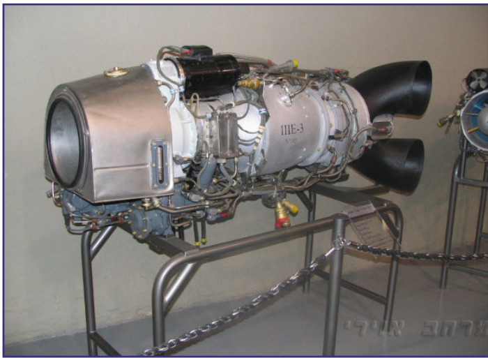
מנוע טורמו-מסוק סופר פרלון.
