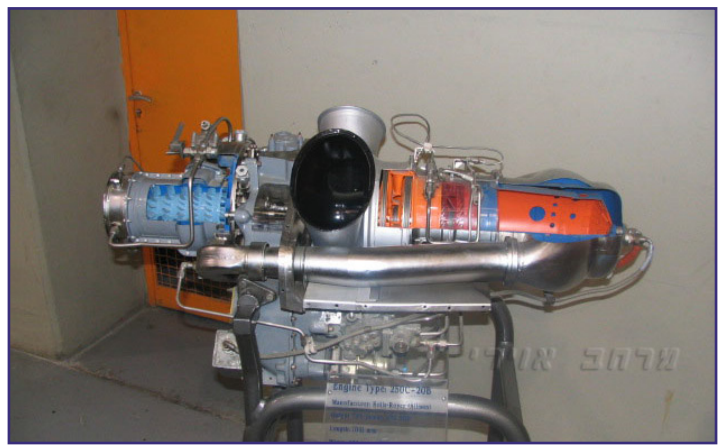
חתך מנוע אליסון -250 מסוק בל 206.
